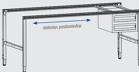
3. Schritt: Trägerpaar
