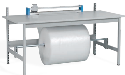
Untertisch-Achsablage mit Hintertisch-Schneidgerät
