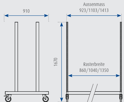
Transportwagen 4
