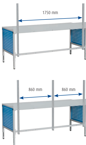
Rasterbreiten bei einer Tischbreite von 2000 mm
