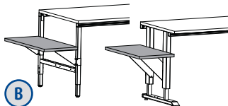
Seitlicher Ablageboden zu ERGO-Basic (Seite 664)/ERGO-Vario Plus (Seite 676)
