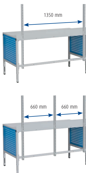
Rasterbreiten bei einer Tischbreite von 1600 mm
